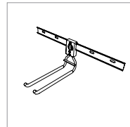
Gerader Werkzeughaken B:70 mm T:262 mm H:151 mm 4700085 23,40
