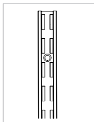
Verlängerung Hängeschiene B:25 mm T:27 mm H:1148 mm
