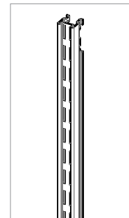
Hängeschiene B:25 mm T:27 mm H:1020-2172 mm
