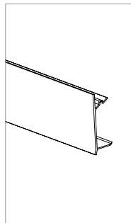
Tragleistenabdeckung B:581 mm T:15 mm H:48 mm
